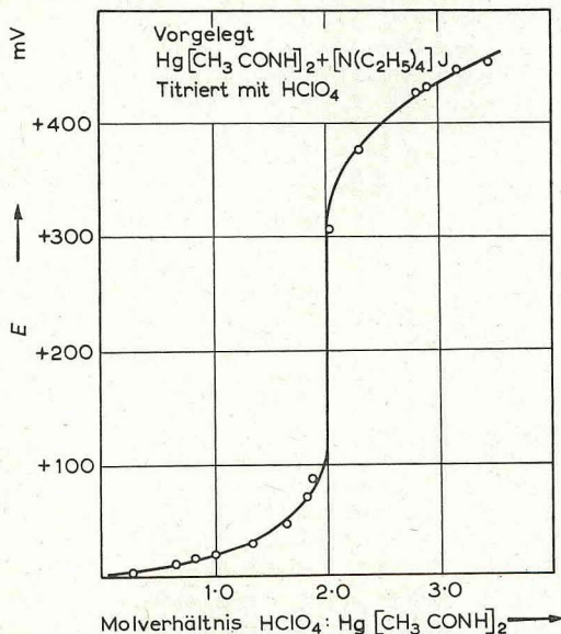
ABB. 3.—Potentiometrische Titration des durch doppelte Umsetzung aus \text{Hg}[\text{CH}_3\text{CONH}_2]_2 und [\text{N}(\text{C}_2\text{H}_5)_4]\text{J} in Lösung erhaltenen Tetraäthylammoniumacetamid mit \text{HClO}_4 .
