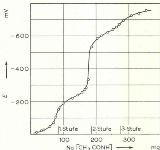
ABB. 4.—Potentiometrische Stufentitration verschieden starker Säuren mit Na-Acetamid.
